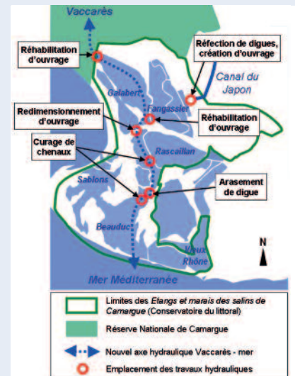
Carte des travaux hydrauliques prévus dans le cadre du programme LIFE + MC-SALT.
